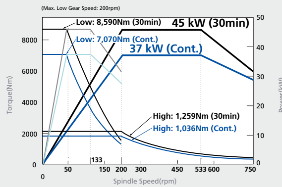
Hi-TECH 850BB+ (Main Spindle)
